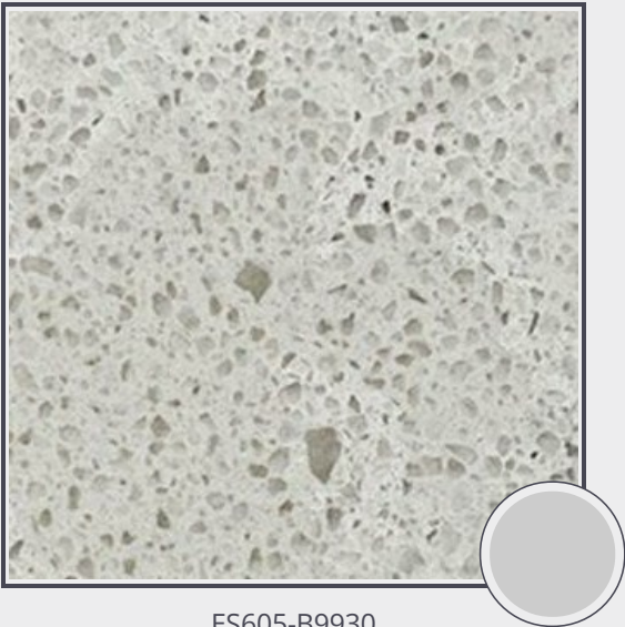
ES605-B9930
